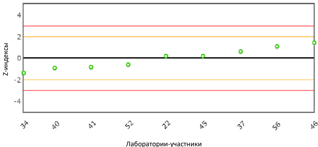
Рис. 30 Распределение z-индексов для показателя «Давление насыщенных паров, кПа»
