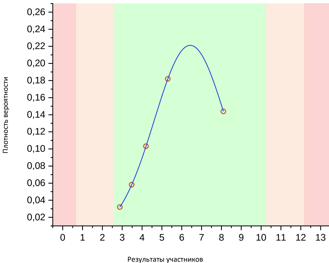
Рис. 2 Нормальное распределение по показателю «Фракционный состав: начало кипения, °С»
