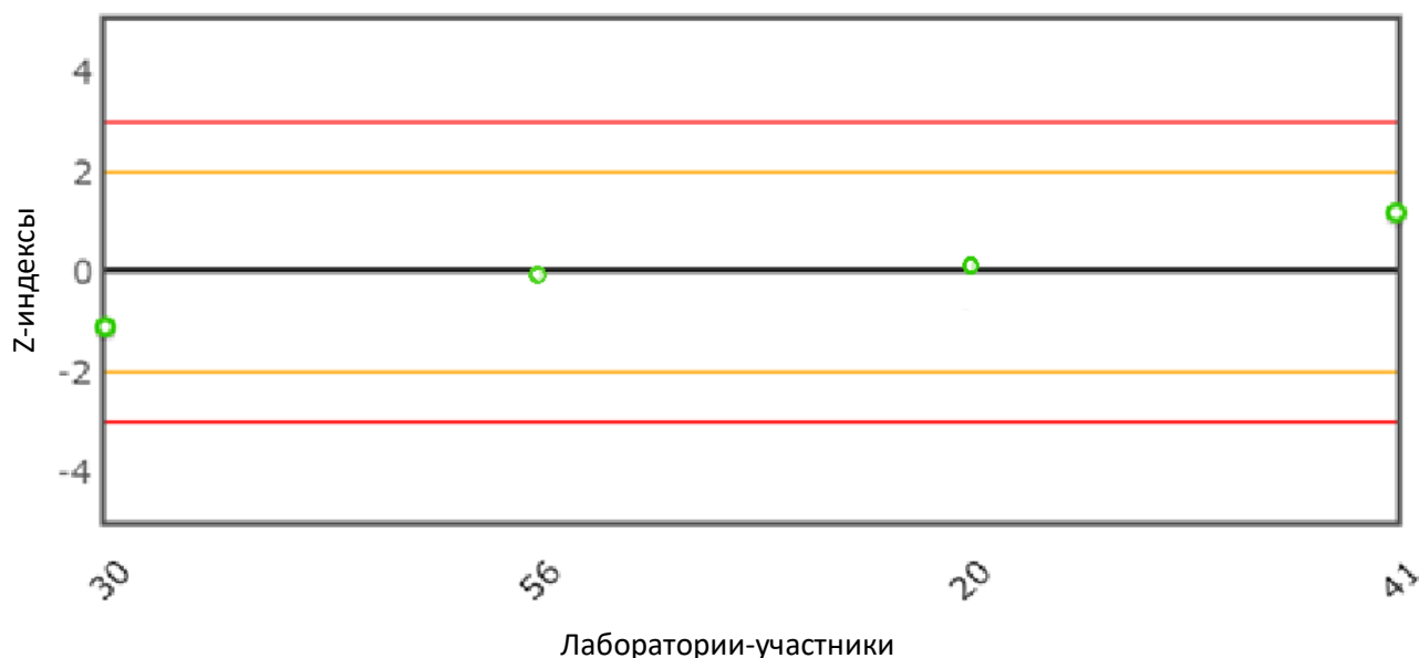
Рис. 24 Распределение z-индексов для показателя «Октановое число (моторный метод), ед.»
