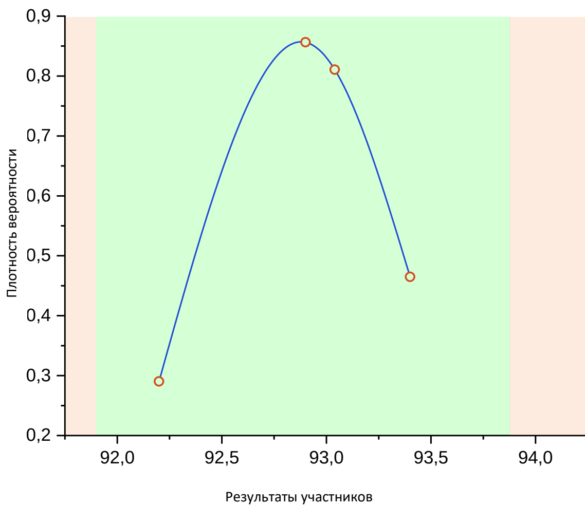
Рис. 27 Нормальное распределение по показателю «Октановое число (исследовательский метод), ед.»
