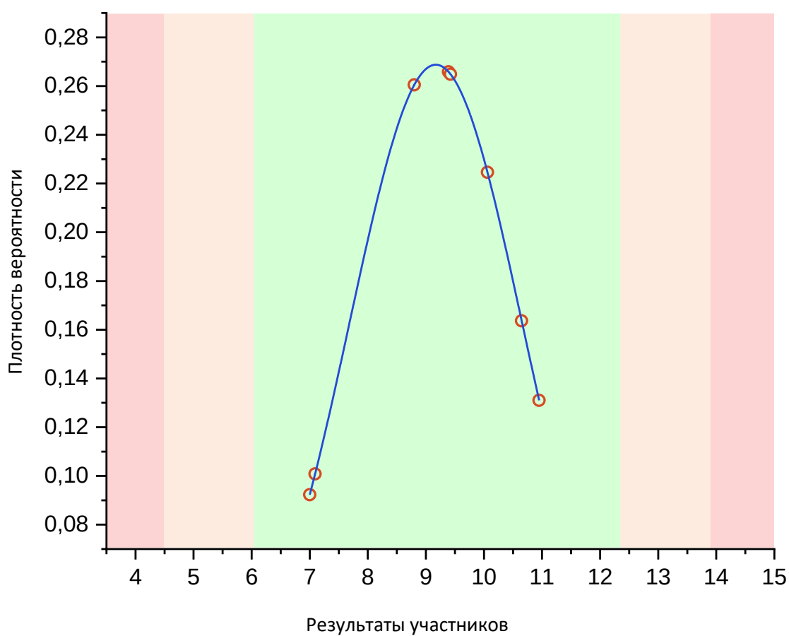
Рис. 20 Нормальное распределение по показателю «Объемная доля олефиновых углеводородов, %»
