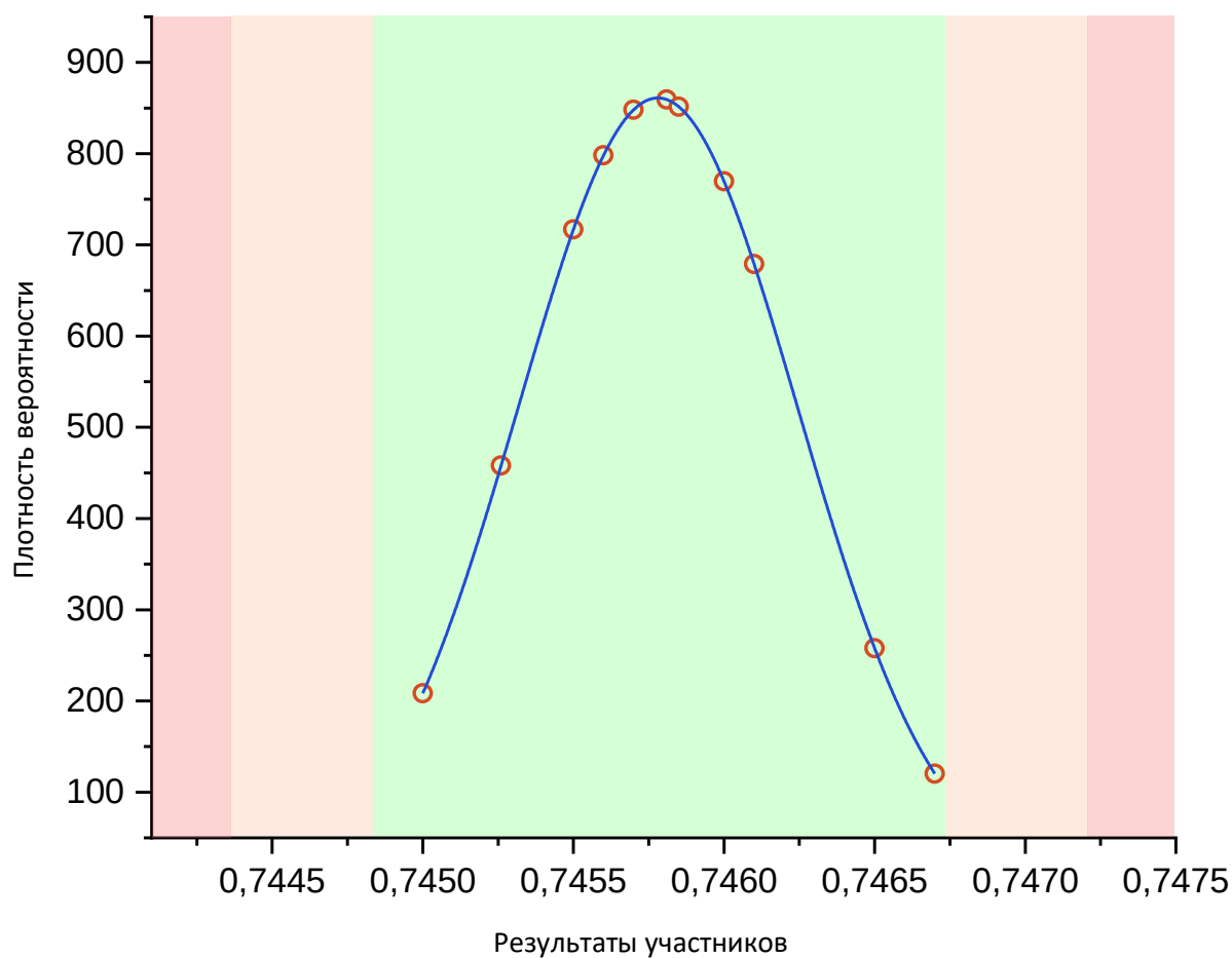
Рис. 18 Нормальное распределение по показателю «Плотность при 15 °С, г/см 3 »
