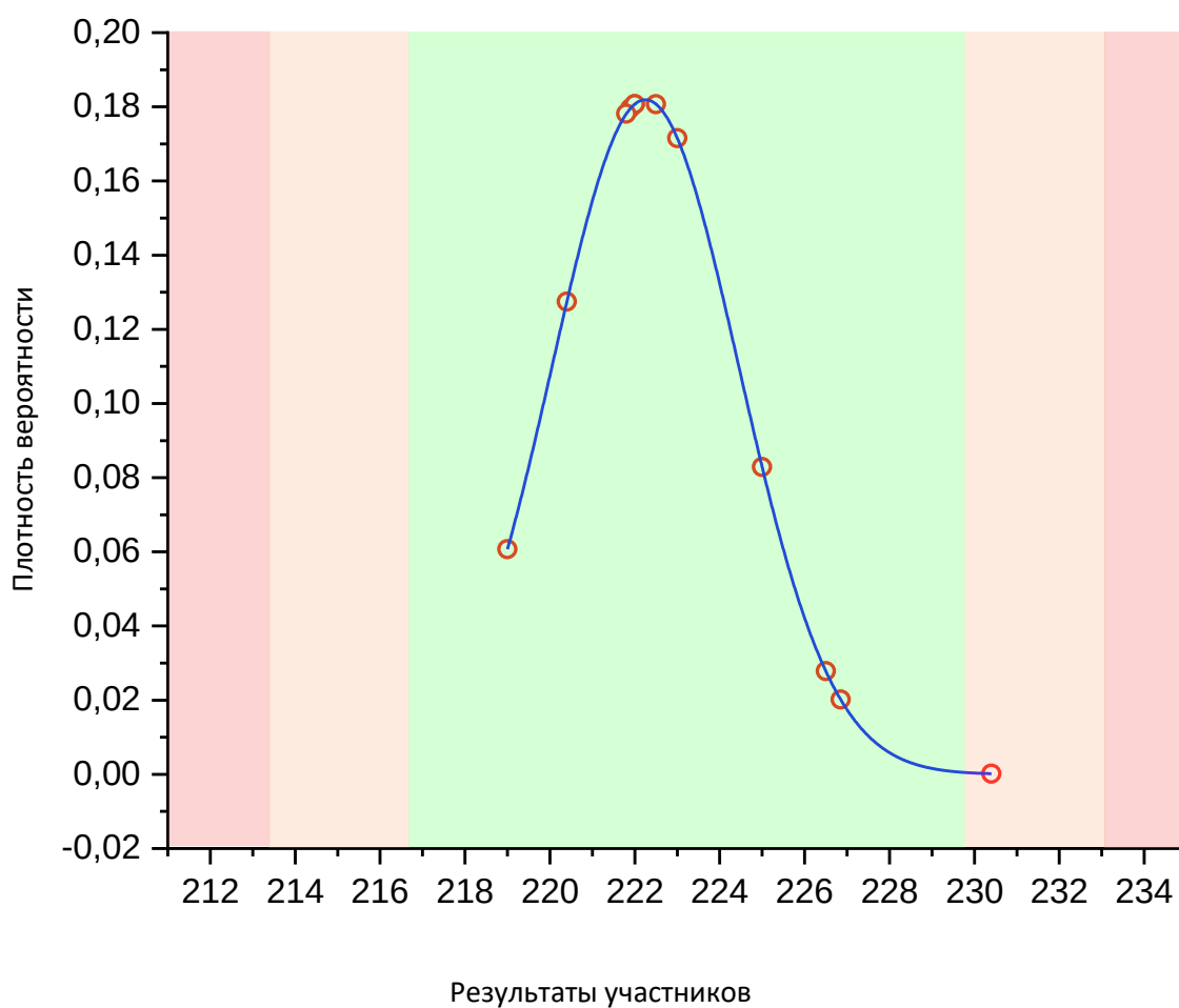
Рис. 10 Нормальное распределение по показателю «Фракционный состав: конец кипения, °C»
