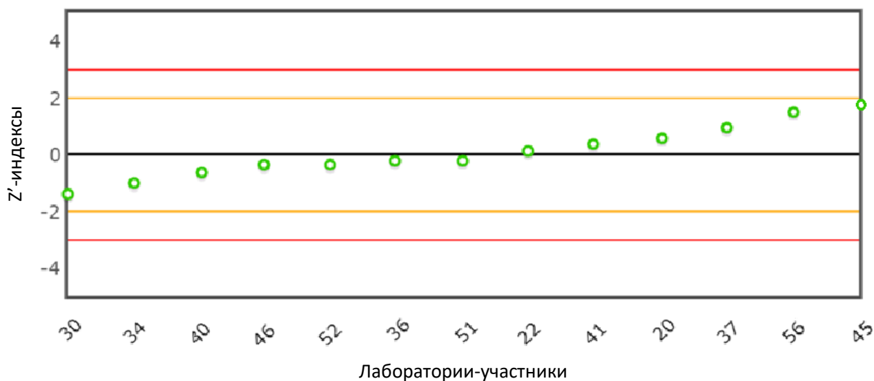
Рис. 17 Распределение z'-индексов для показателя «Плотность при 15 °С, г/см³»
