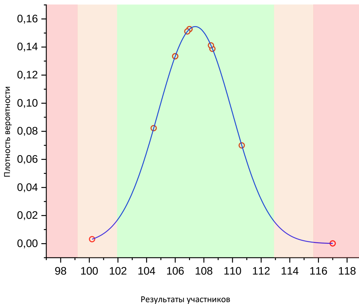
Рис. 6 Нормальное распределение по показателю «Фракционный состав: 50% отгон, °С»
