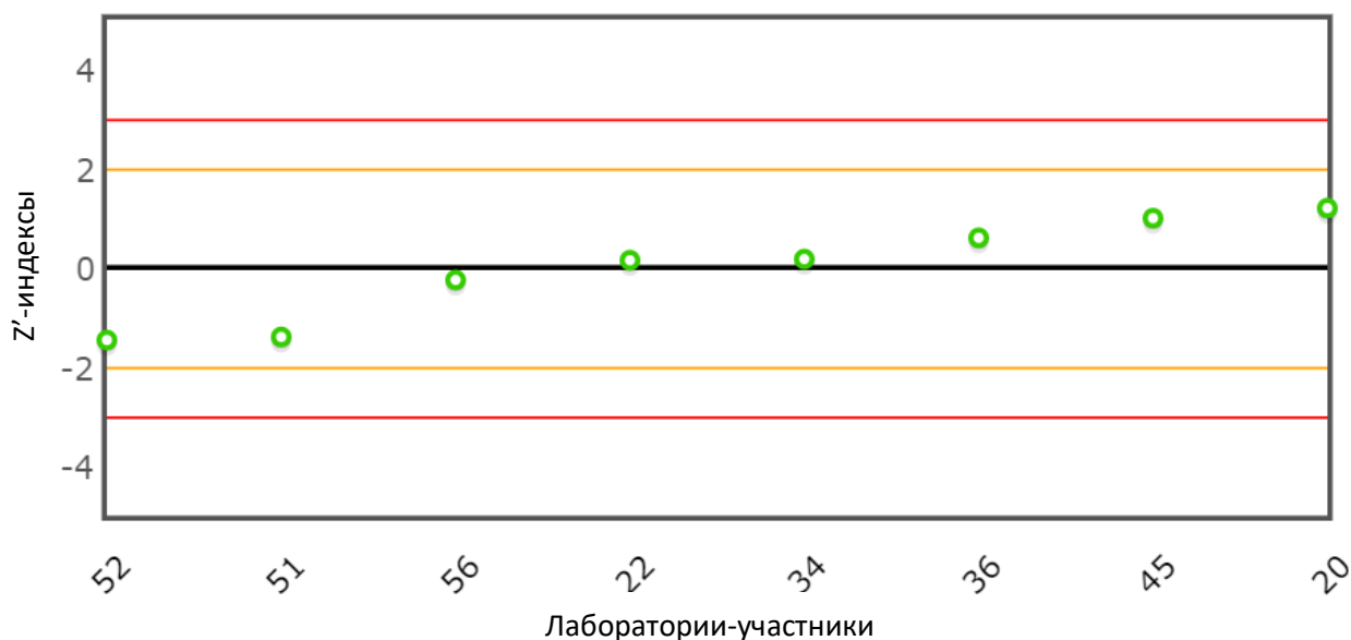
Рис. 19 Распределение z'-индексов для показателя «Объемная доля олефиновых углеводородов, %»
