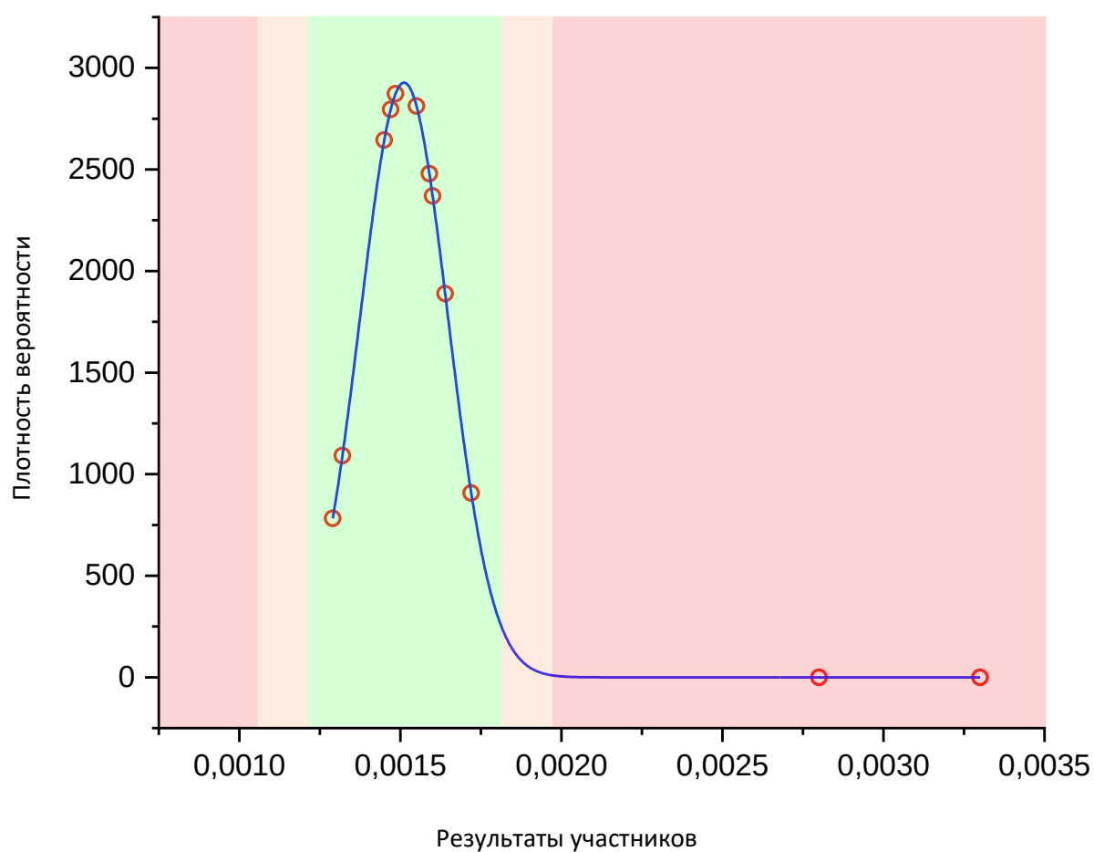
Рис. 12 Нормальное распределение по показателю «Массовая доля серы, %»
