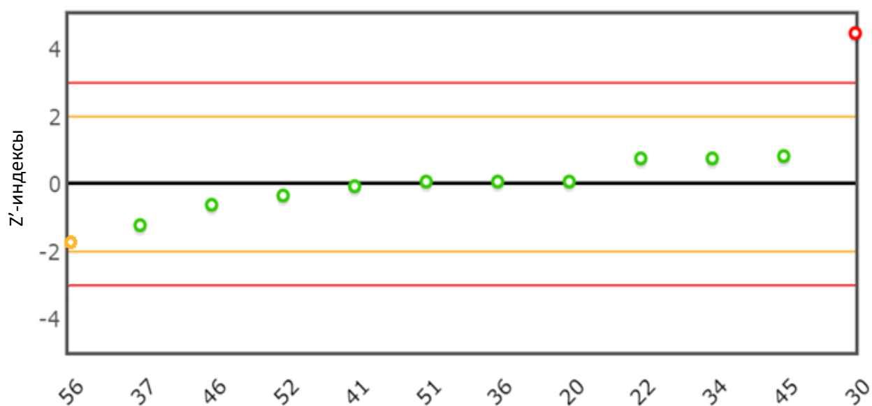
Рис. 3 Распределение z'-индексов для показателя «Фракционный состав: 10% отгон, °С»
