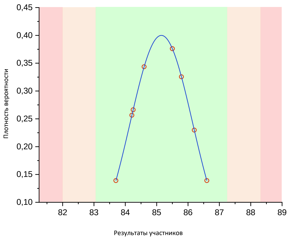
Рис. 31 Нормальное распределение по показателю «Давление насыщенных паров, кПа»
