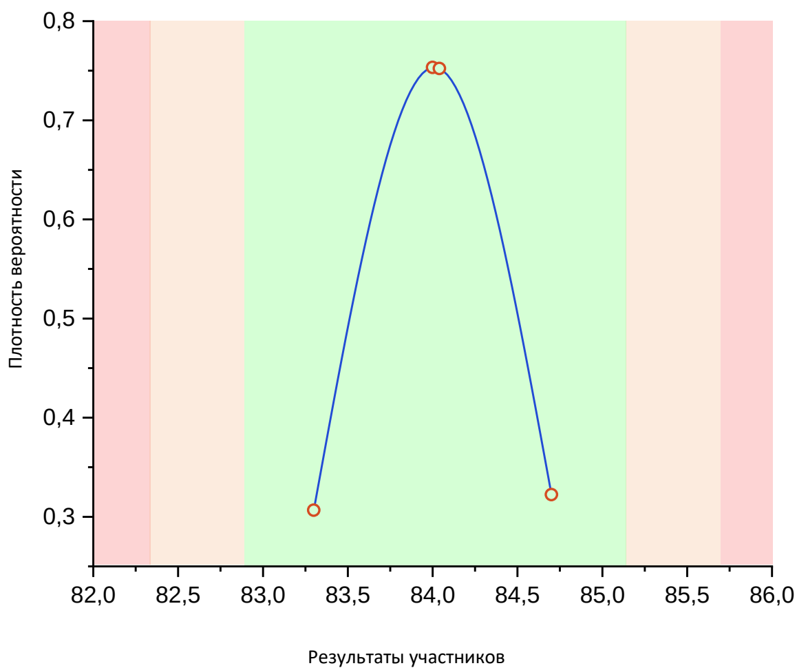
Рис. 25 Нормальное распределение по показателю «Октановое число (моторный метод), ед.»
