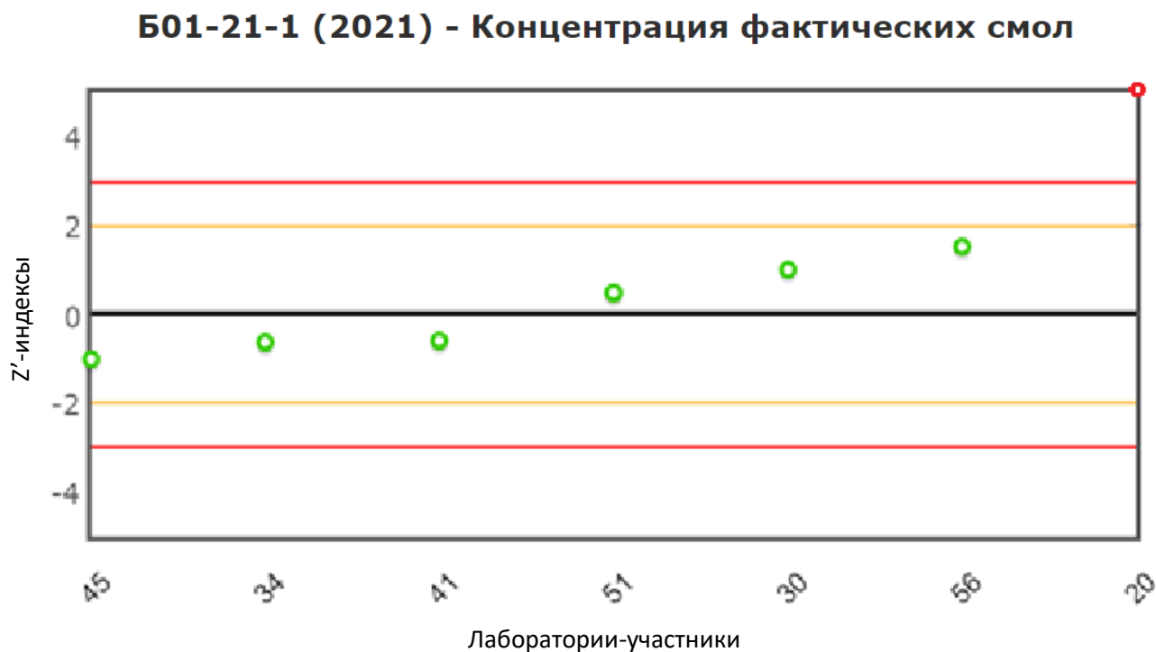
Рис. 15 Распределение z'-индексов для показателя «Концентрация фактических смол, мг/100 см 3 »
