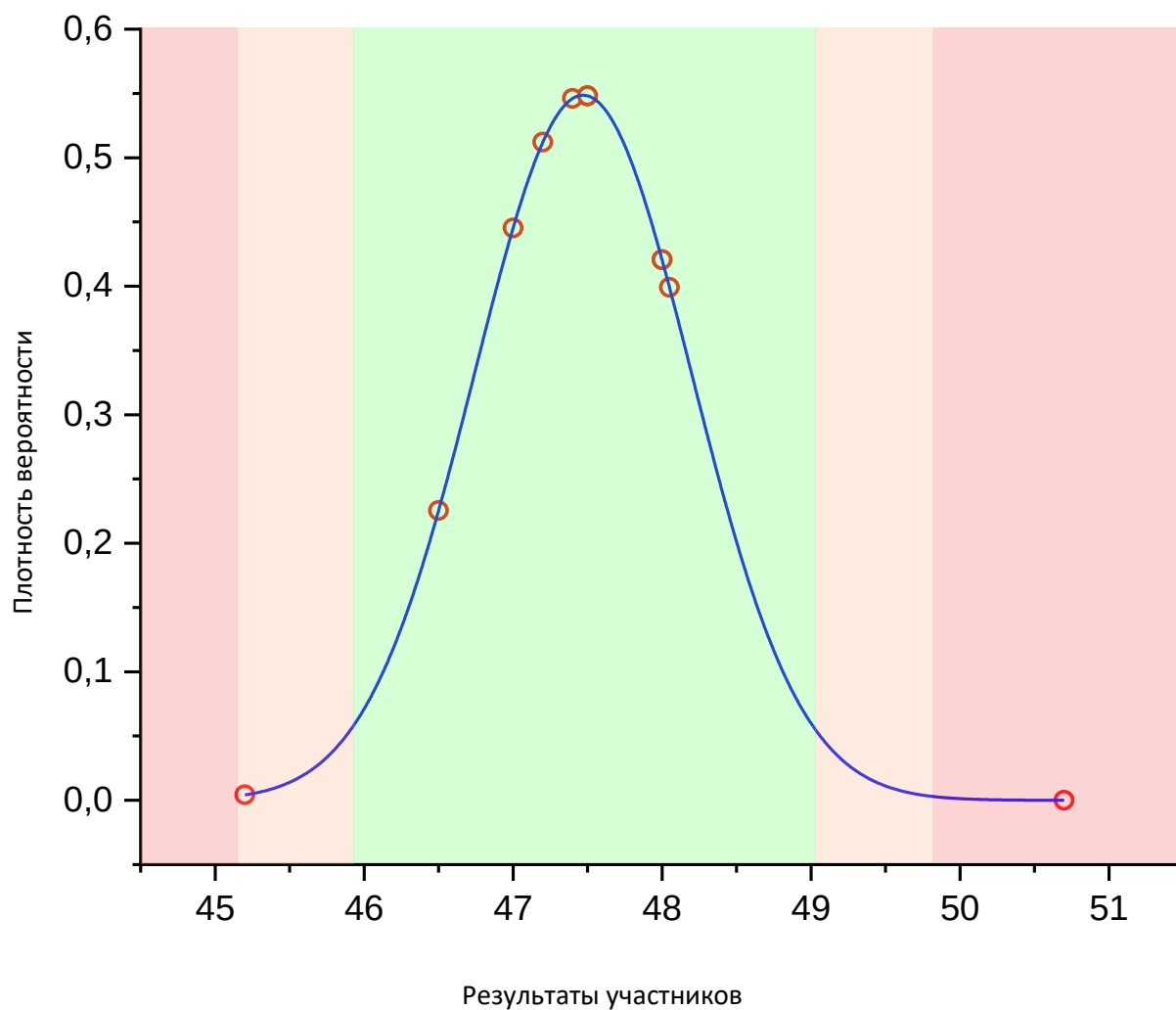
Рис. 4 Нормальное распределение по показателю «Фракционный состав: 10% отгон, °С»
