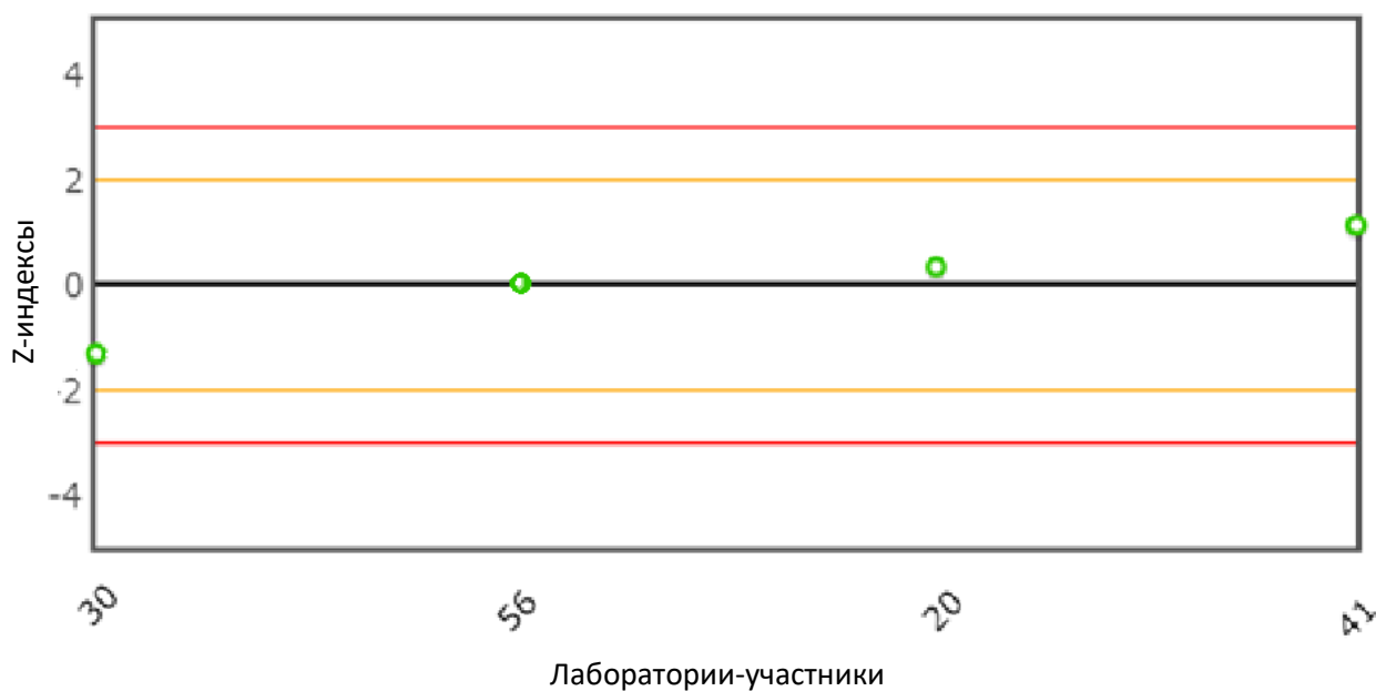
Рис. 26 Распределение z-индексов для показателя «Октановое число (исследовательский метод), ед.»
