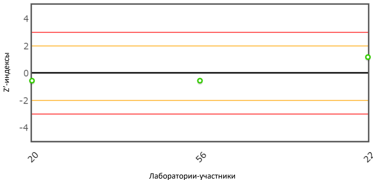
Рис. 23 Распределение z'-индексов для показателя «Объемная доля монометиланилина, %»
