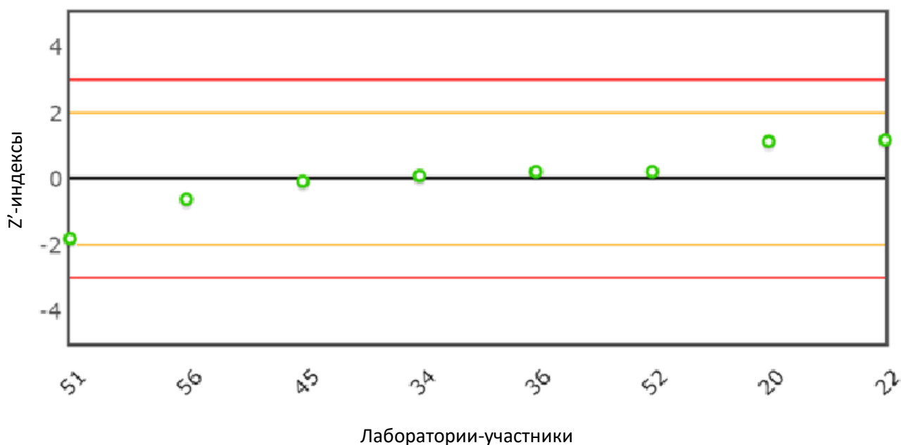
Рис. 13 Распределение z'-индексов для показателя «Объемная доля бензола, %»
