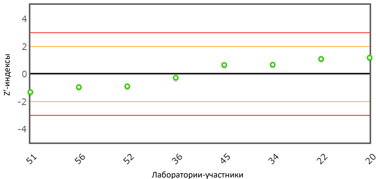
Рис. 21 Распределение z'-индексов для показателя «Объемная доля ароматических углеводородов, %»
