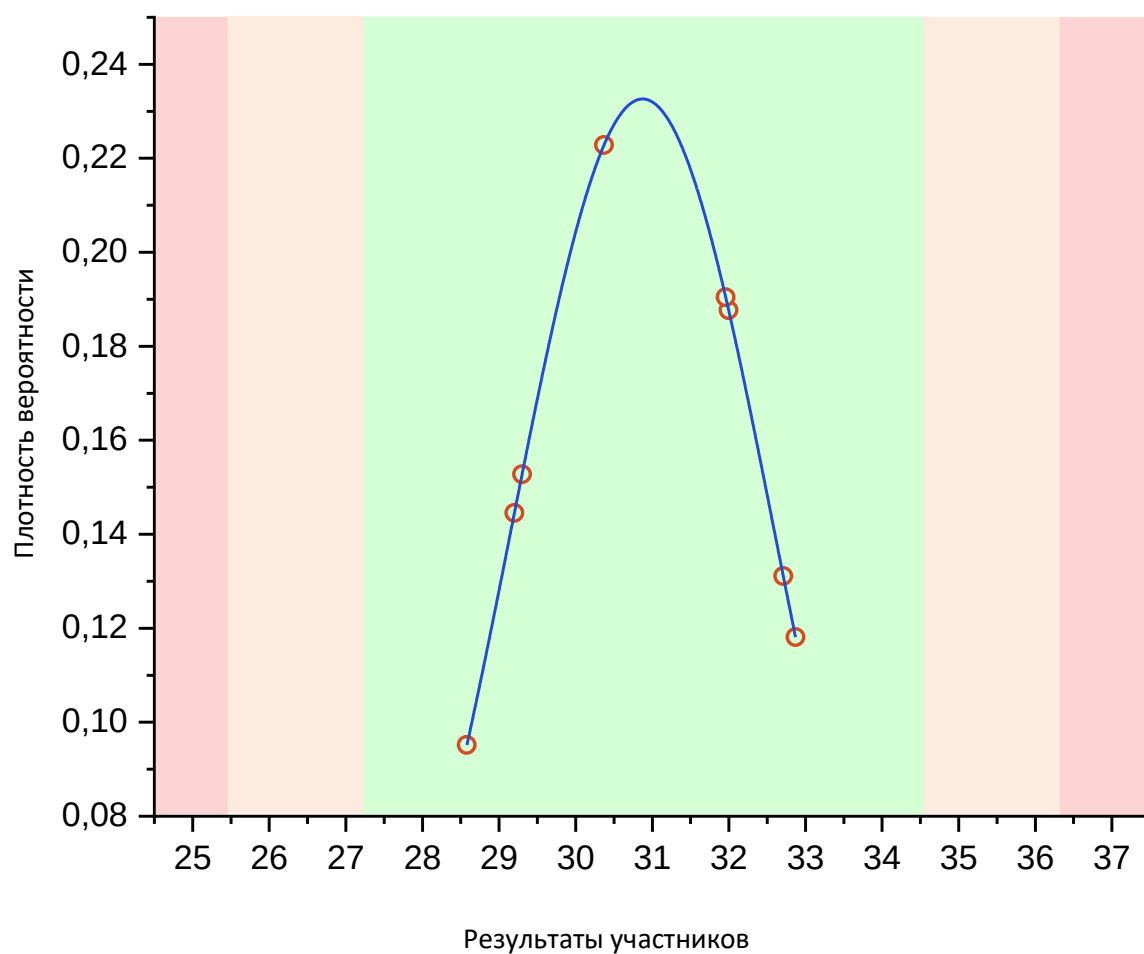
Рис. 22 Нормальное распределение по показателю «Объемная доля ароматических углеводородов, %»
