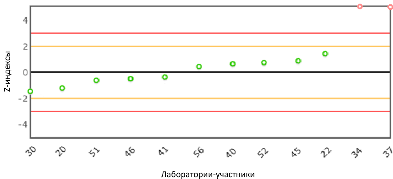
Рис. 11 Распределение z-индексов для показателя «Массовая доля серы, %»
