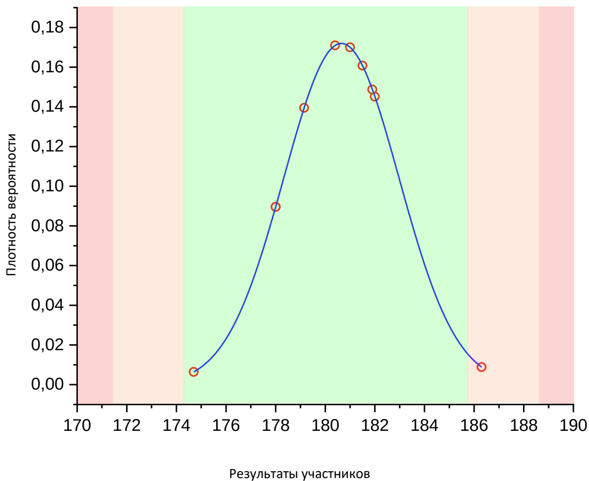
Рис. 8 Нормальное распределение по показателю «Фракционный состав: 90% отгон, °С»
