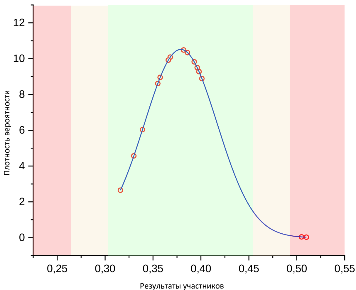
Рис. 12 Нормальное распределение по показателю «Массовая доля серы»
