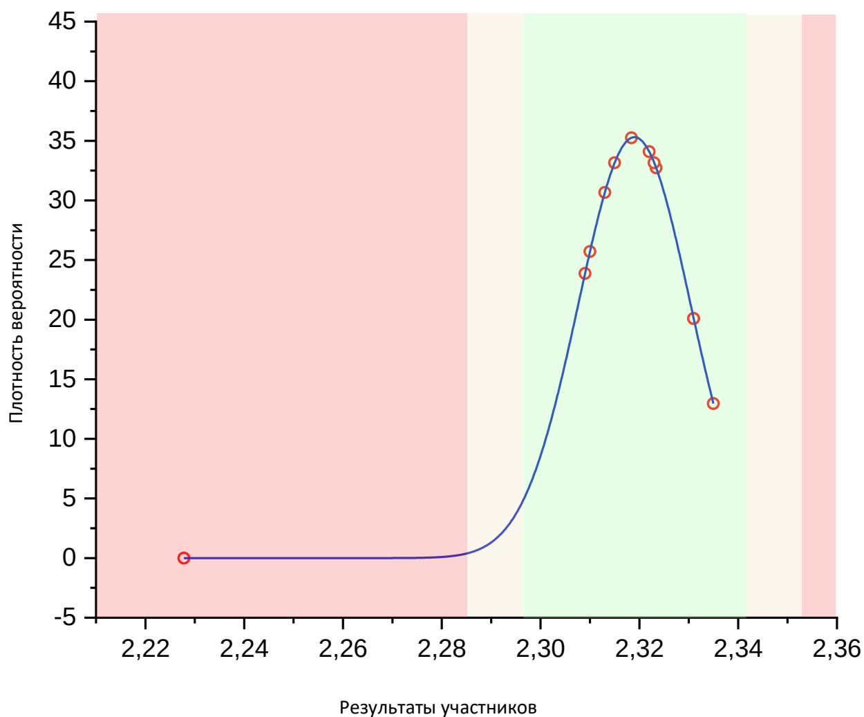
Рис. 6 Нормальное распределение по показателю «Кинематическая вязкость при 20 °С»
