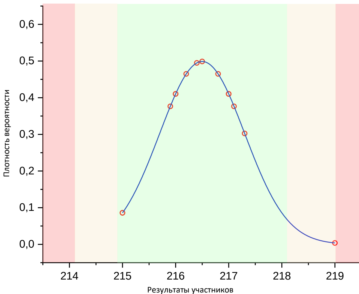
Рис. 8 Нормальное распределение по показателю «Фракционный состав: отгон 50%»
