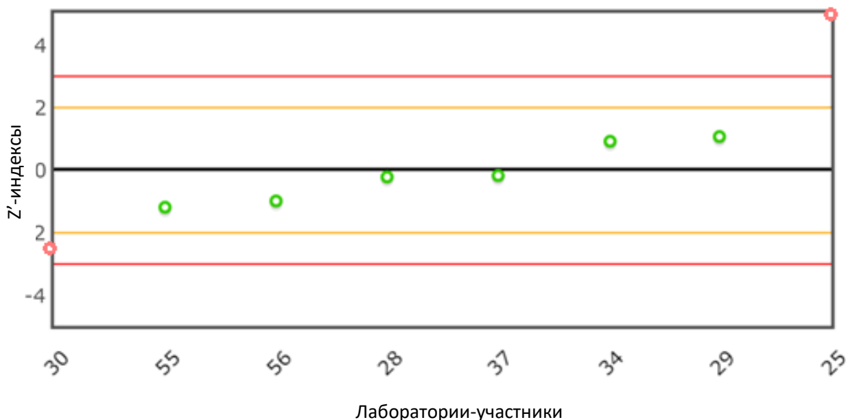
Рис. 1 Распределение z'-индексов для показателя «Кислотность»
