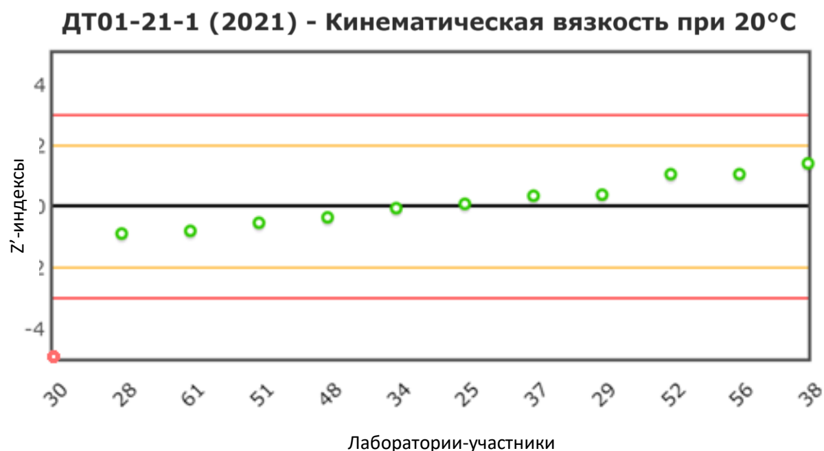
Рис. 5 Распределение z'-индексов для показателя «Кинематическая вязкость при 20 °С»
