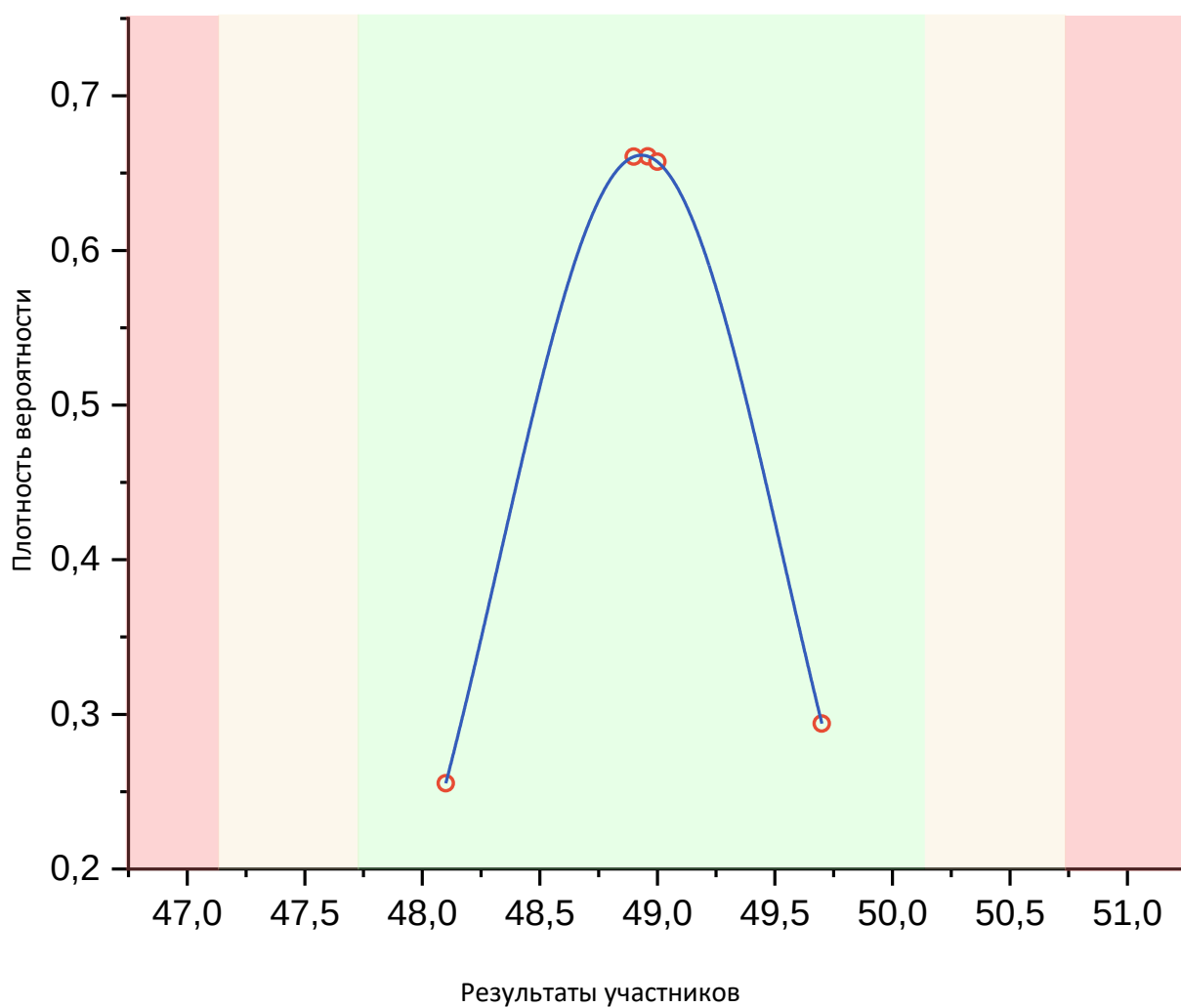
Рис. 29 Нормальное распределение по показателю «Цетановое число»
