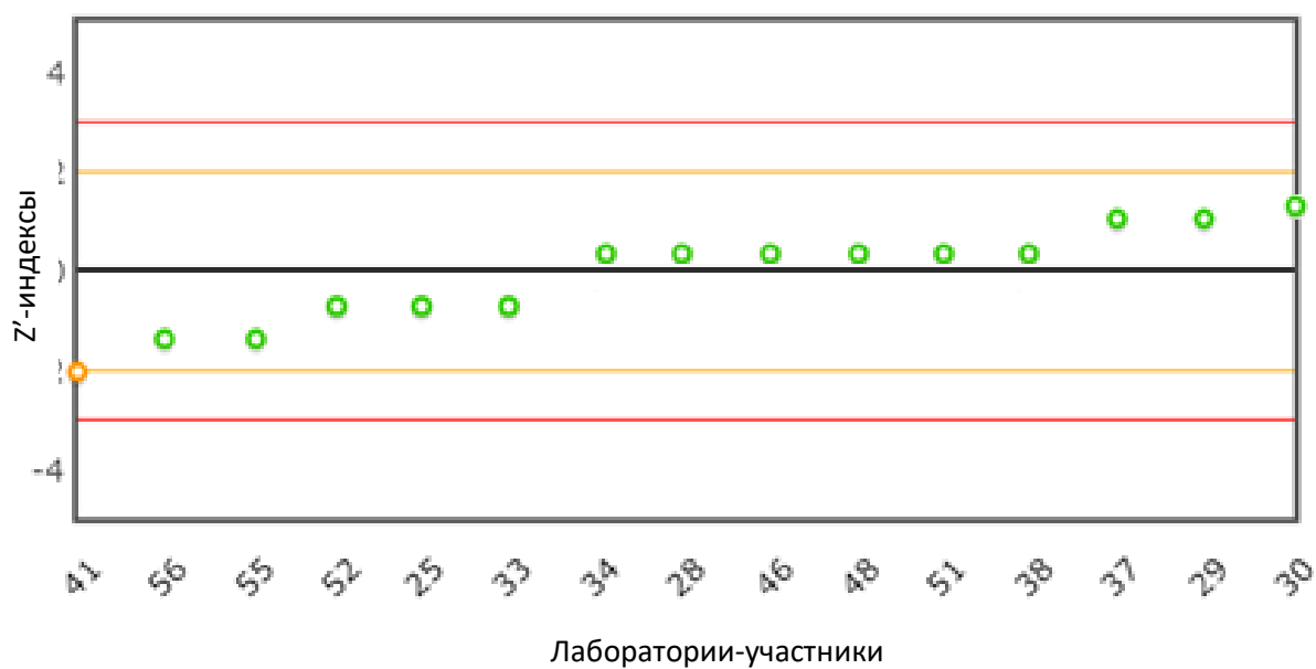
Рис. 23 Распределение z'-индексов для показателя «Температура помутнения»
