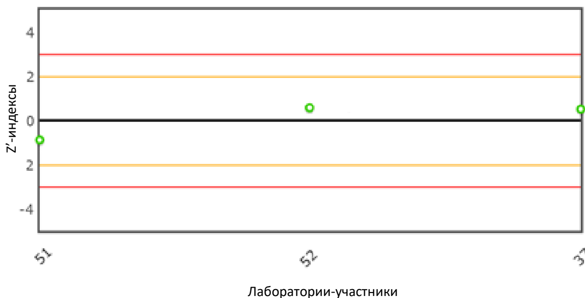
Рис. 27 Распределение z'-индексов для показателя «Коксуемость»
