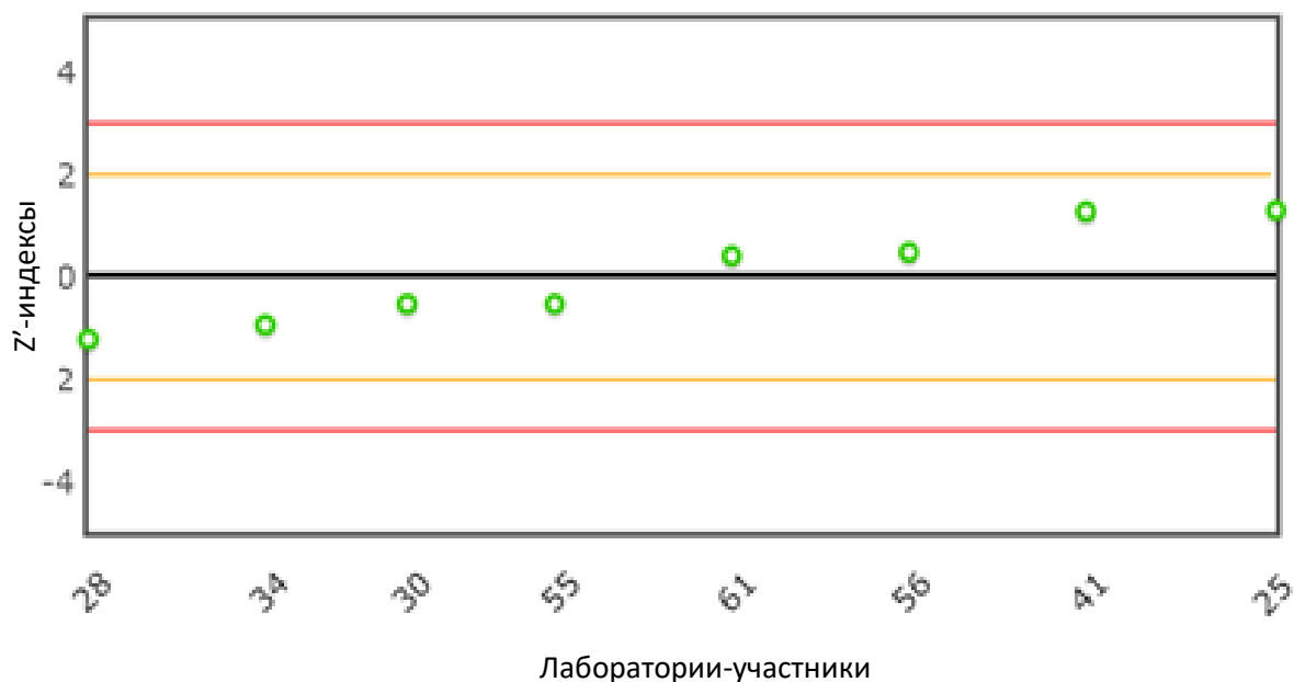
Рис. 17 Распределение z'-индексов для показателя «Температура застывания»
