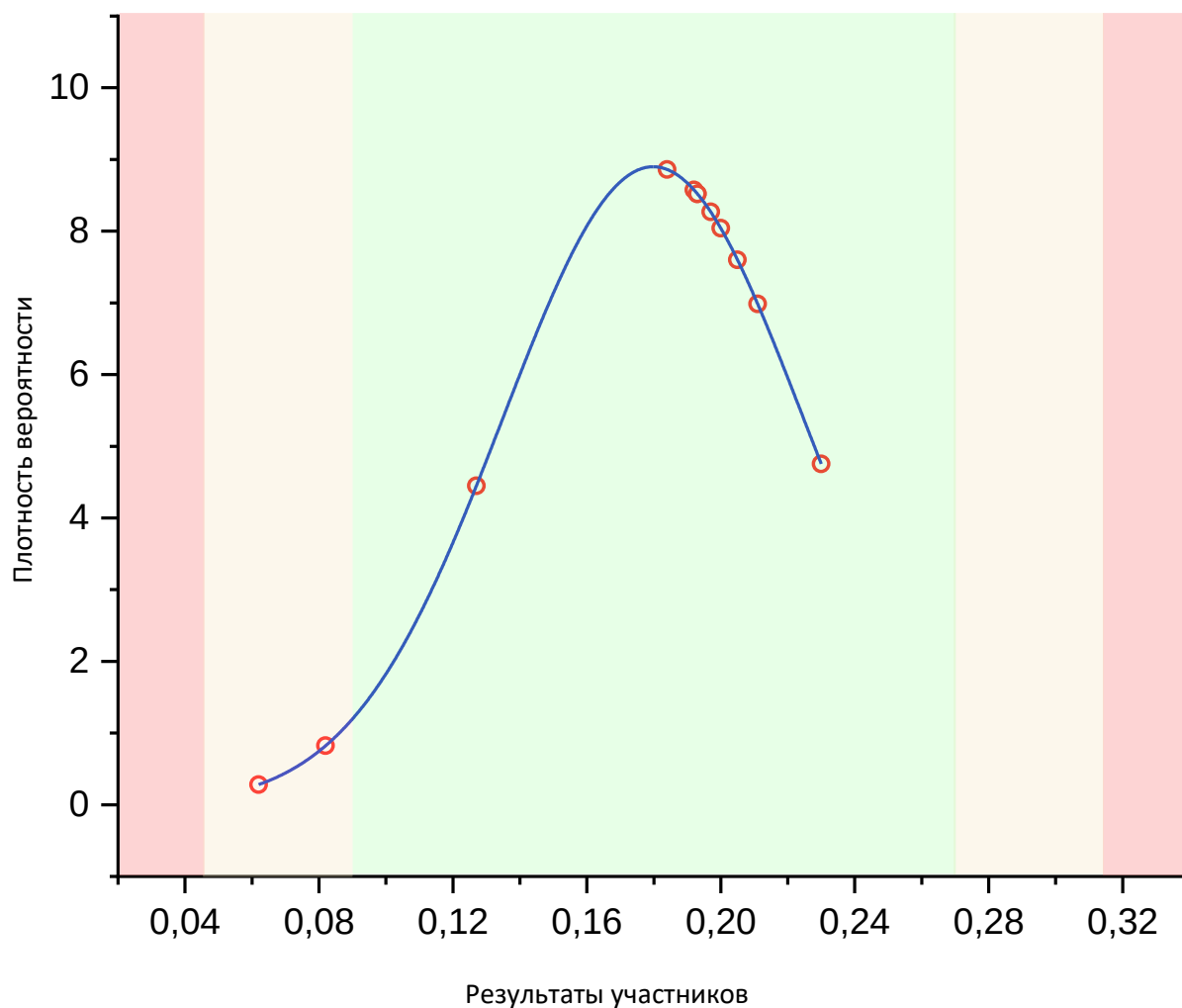
Рис. 22 Нормальное распределение по показателю «Зольность»
