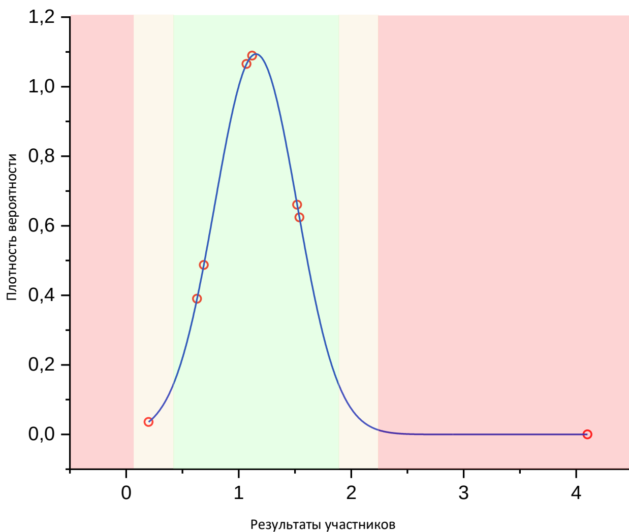
Рис. 2 Нормальное распределение по показателю «Кислотность»
