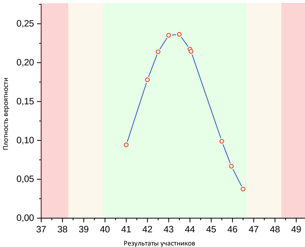
Рис. 14 Нормальное распределение по показателю «Температура вспышки в закрытом тигле»
