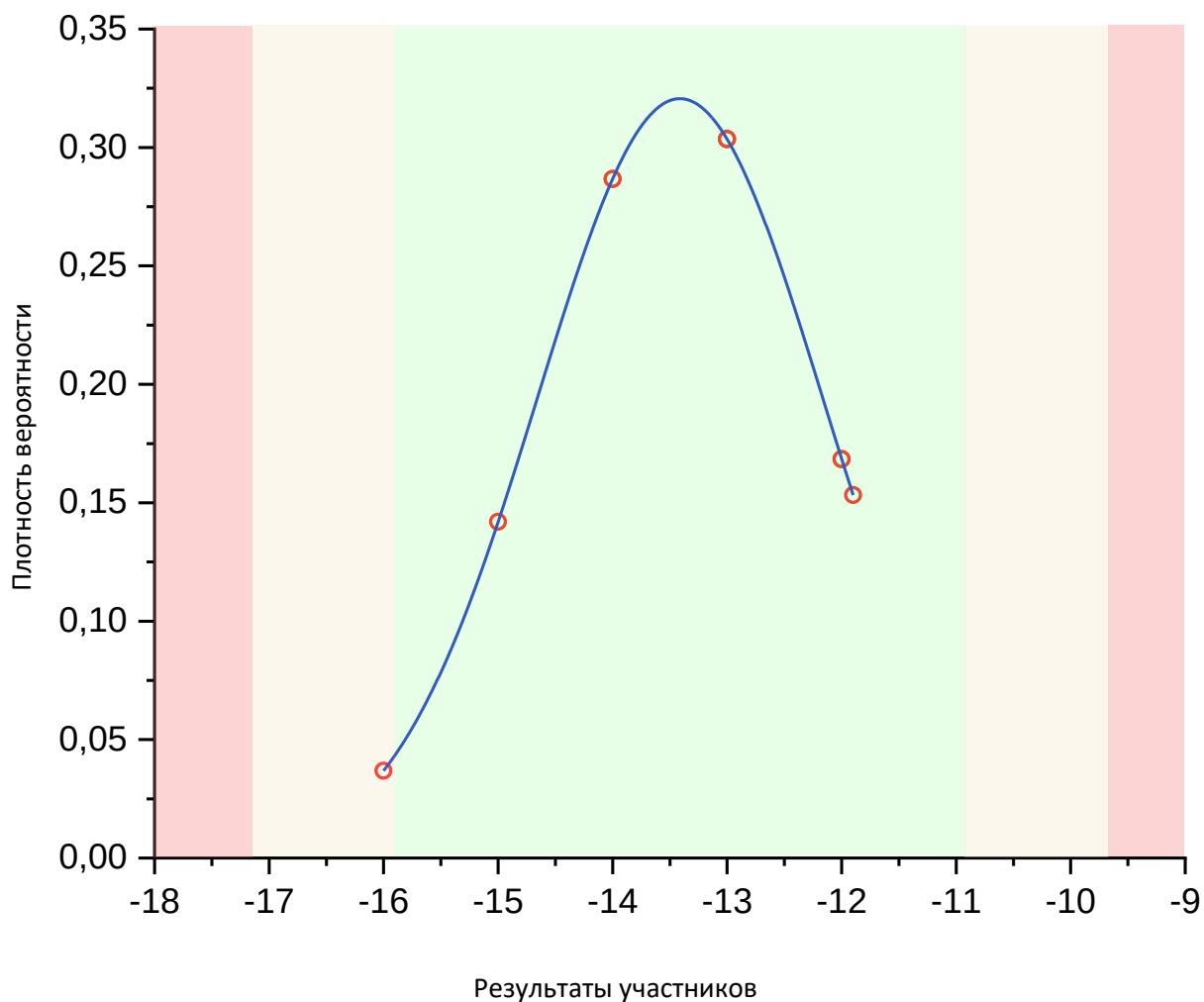
Рис. 24 Нормальное распределение по показателю «Температура помутнения»
