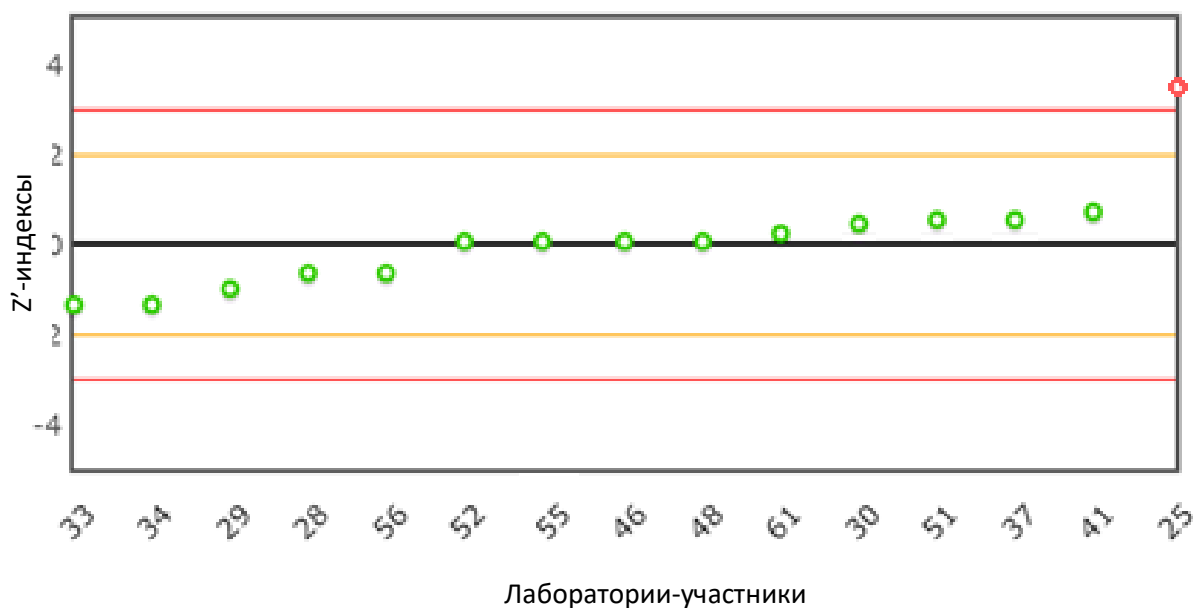
Рис. 15 Распределение z'-индексов для показателя «Предельная температура фильтруемости»
