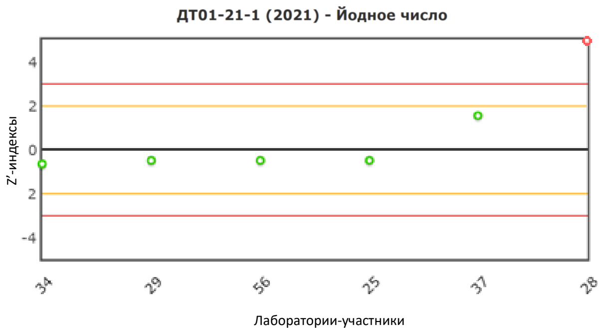
Рис. 19 Распределение z'-индексов для показателя «Йодное число»
