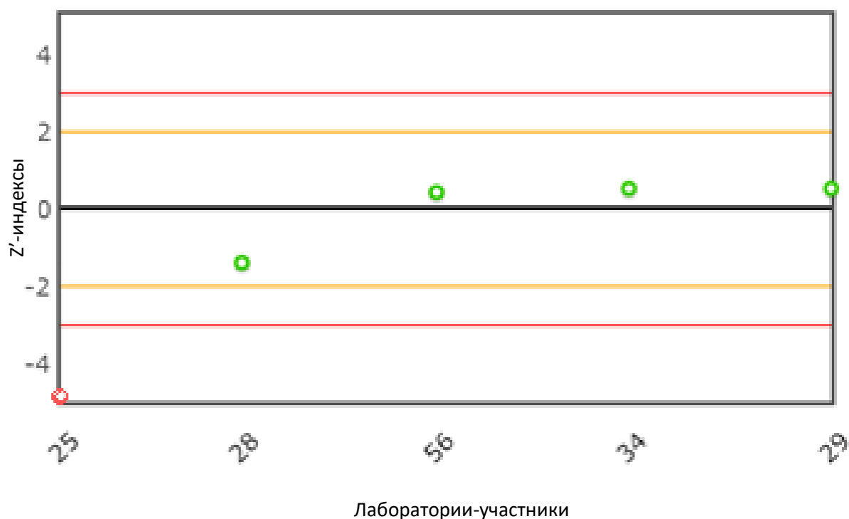
Рис. 25 Распределение z'-индексов для показателя «Коксуемость 10% остатка»
