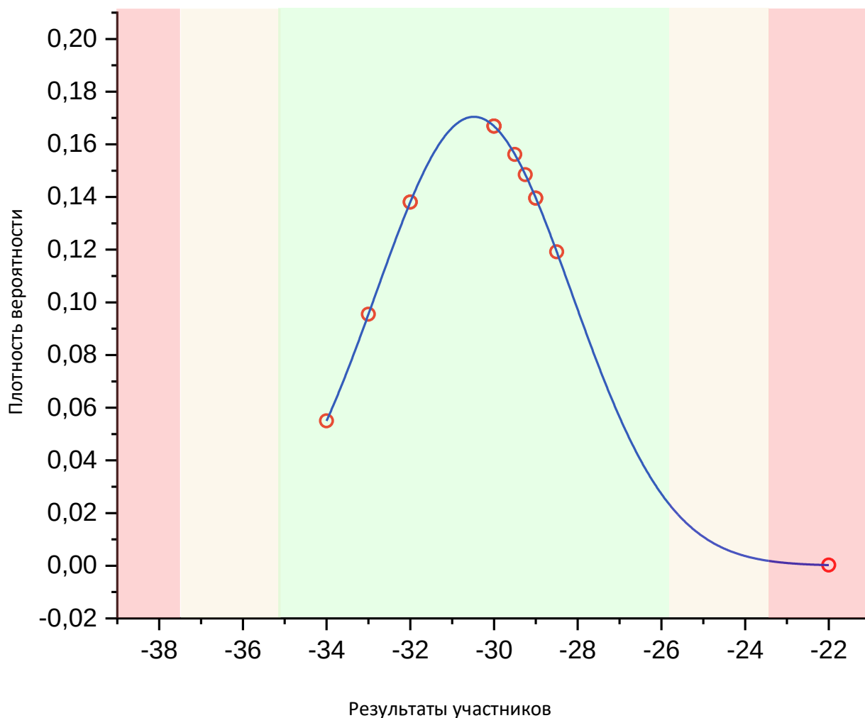
Рис. 16 Нормальное распределение по показателю «Предельная температура фильтруемости»
