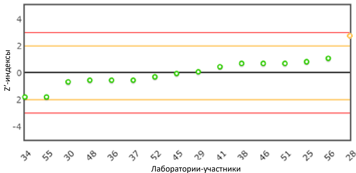
Рис. 7 Распределение z'-индексов для показателя «Фракционный состав: отгон 50%»
