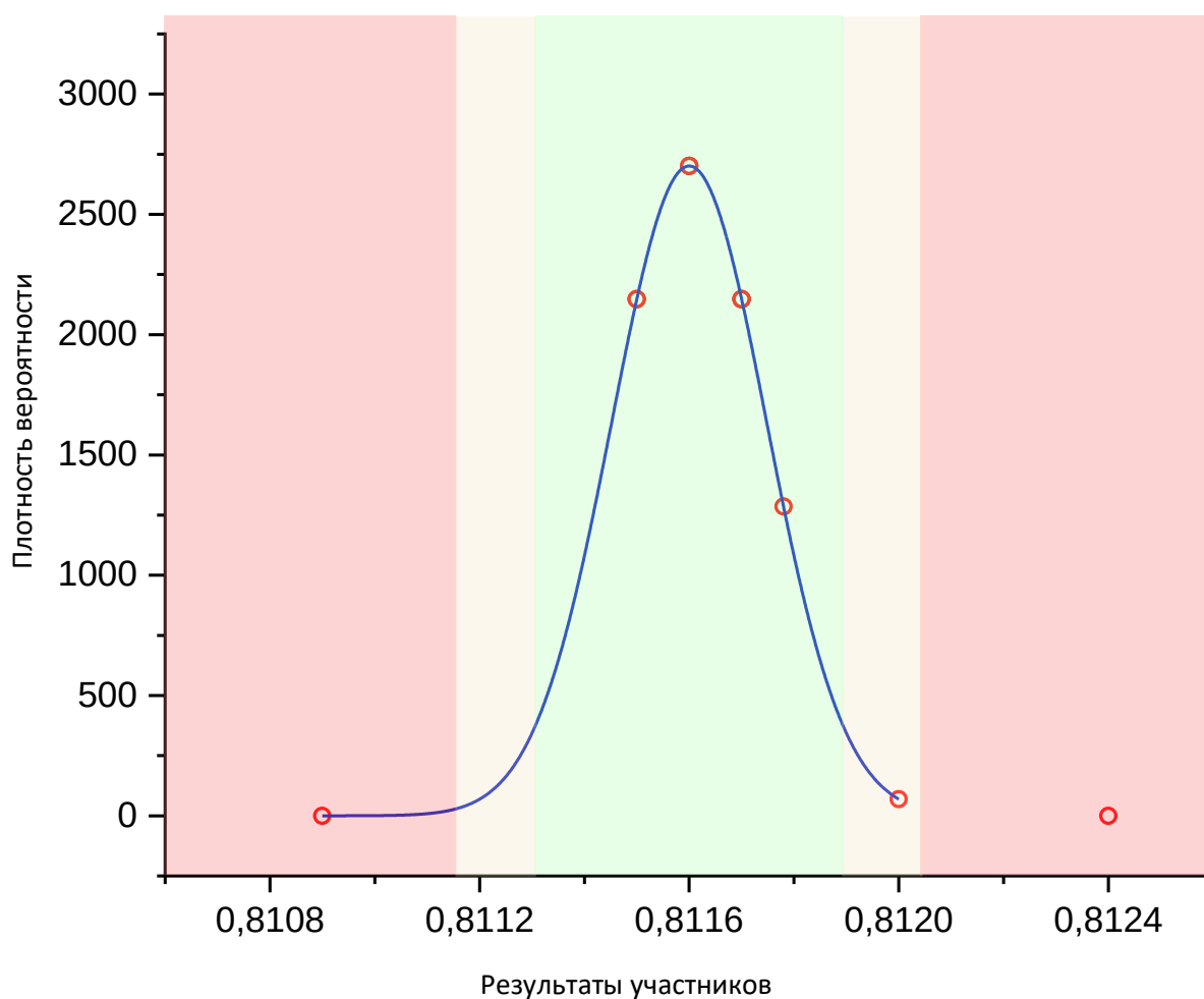
Рис. 4 Нормальное распределение по показателю «Плотность при 15 °С»
