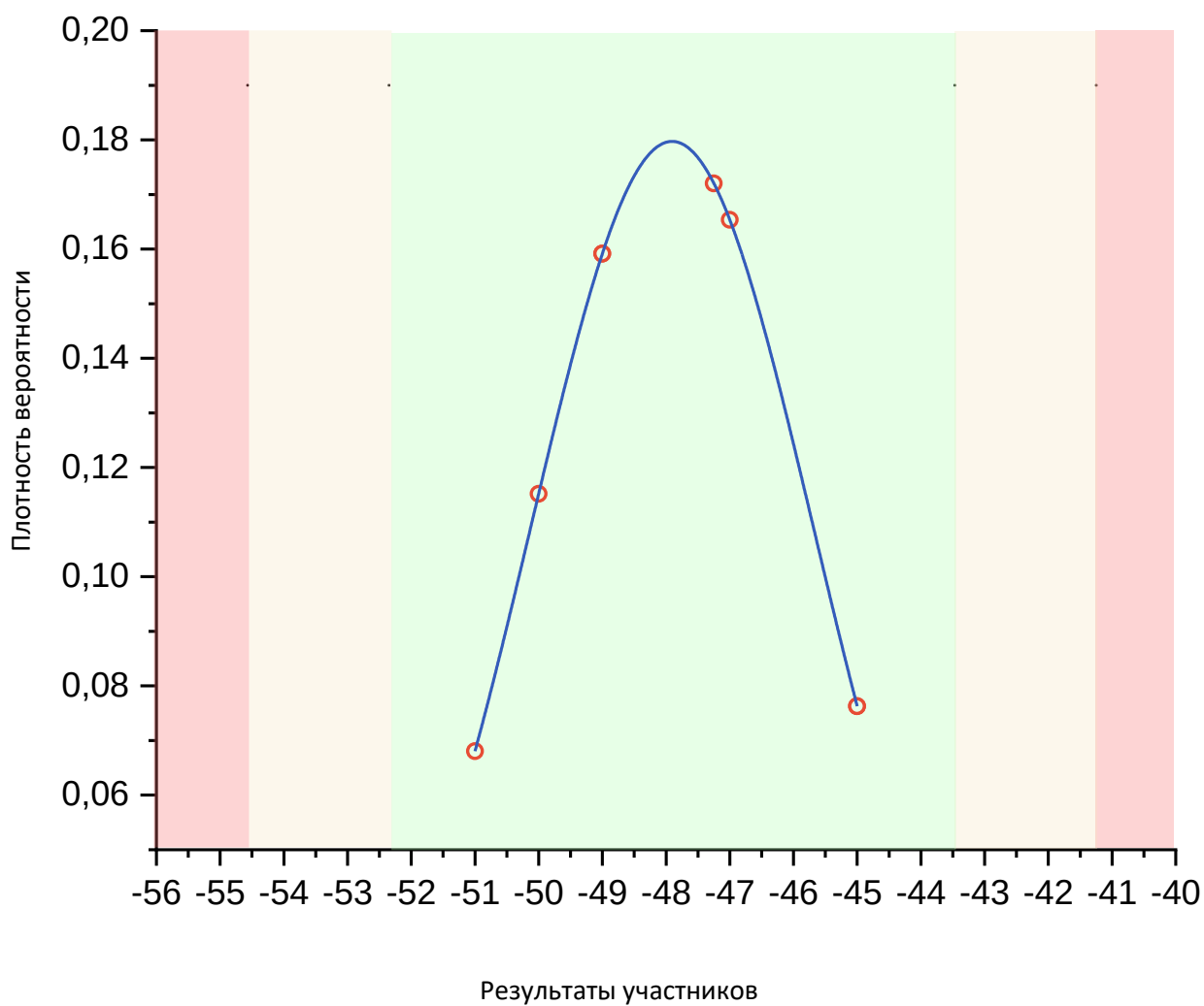
Рис. 18 Нормальное распределение по показателю «Температура застывания»
