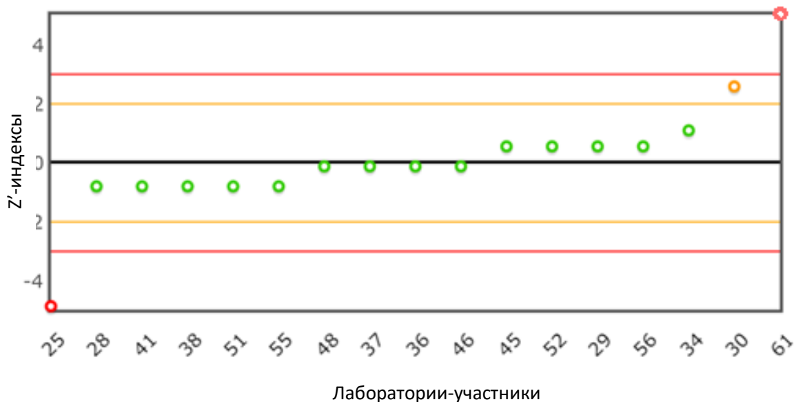
Рис. 3 Распределение z'-индексов для показателя «Плотность при 15 °С»
