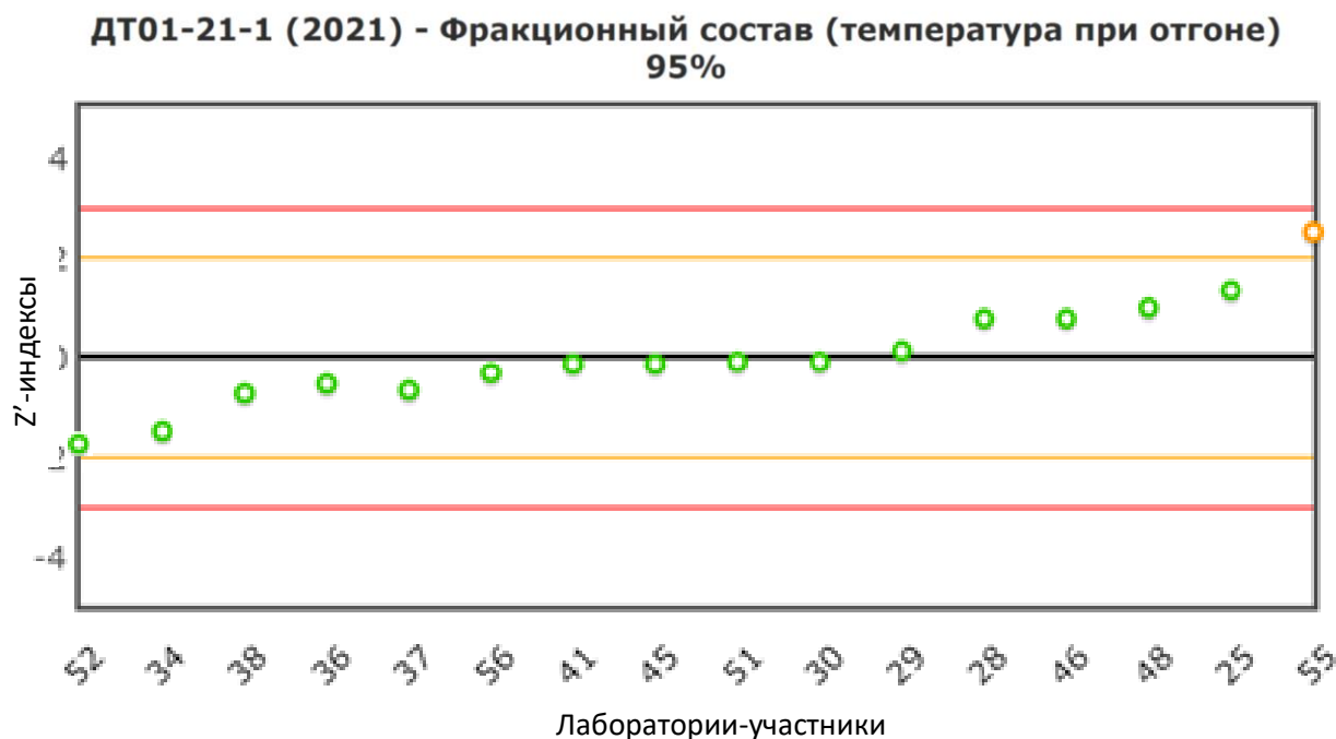
Рис. 9 Распределение z'-индексов для показателя «Фракционный состав: отгон 95%»
