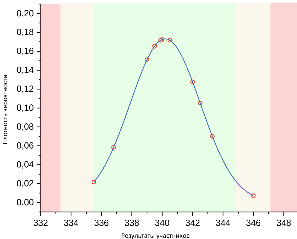
Рис. 10 Нормальное распределение по показателю «Фракционный состав: отгон 95%»
