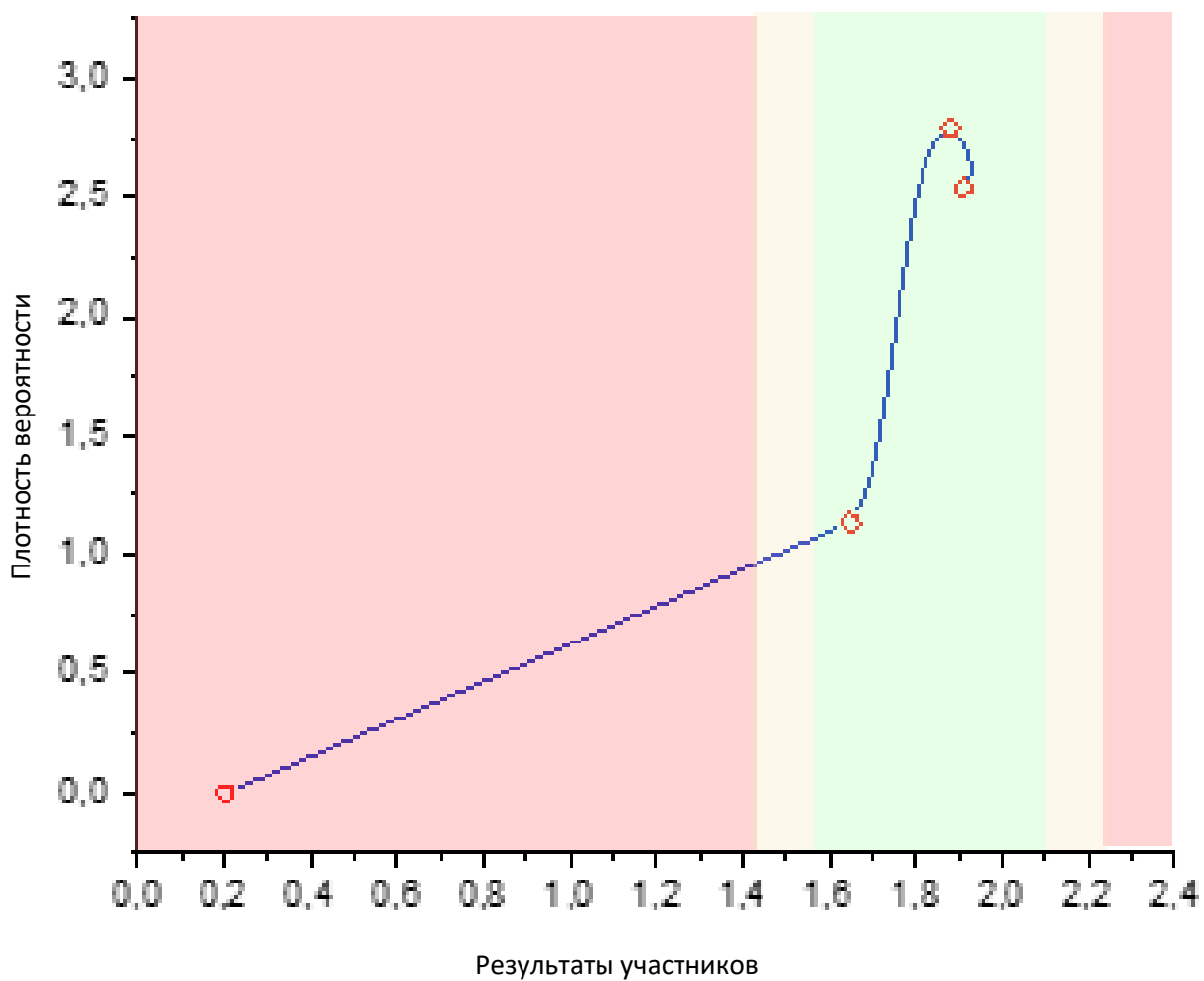
Рис. 26 Нормальное распределение по показателю «Коксуемость 10% остатка»
