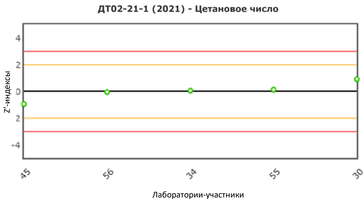
Рис. 28 Распределение z'-индексов для показателя «Цетановое число»
