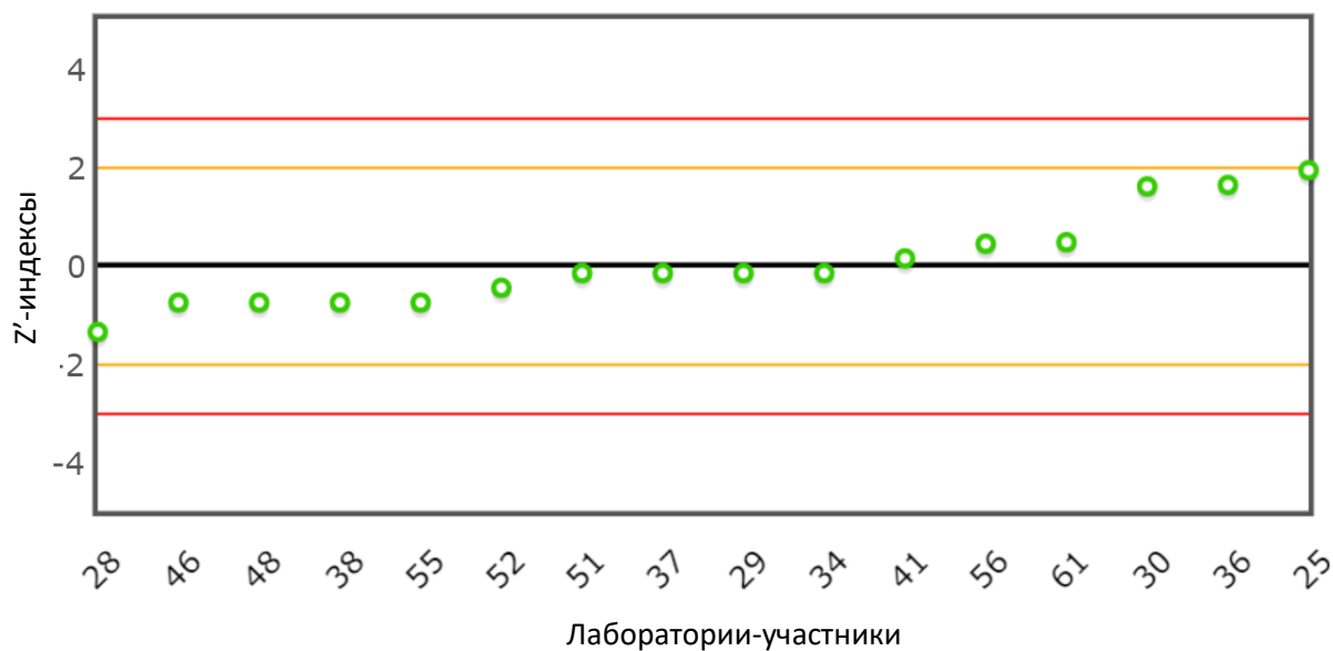
Рис. 13 Распределение z'-индексов для показателя «Температура вспышки в закрытом тигле»
