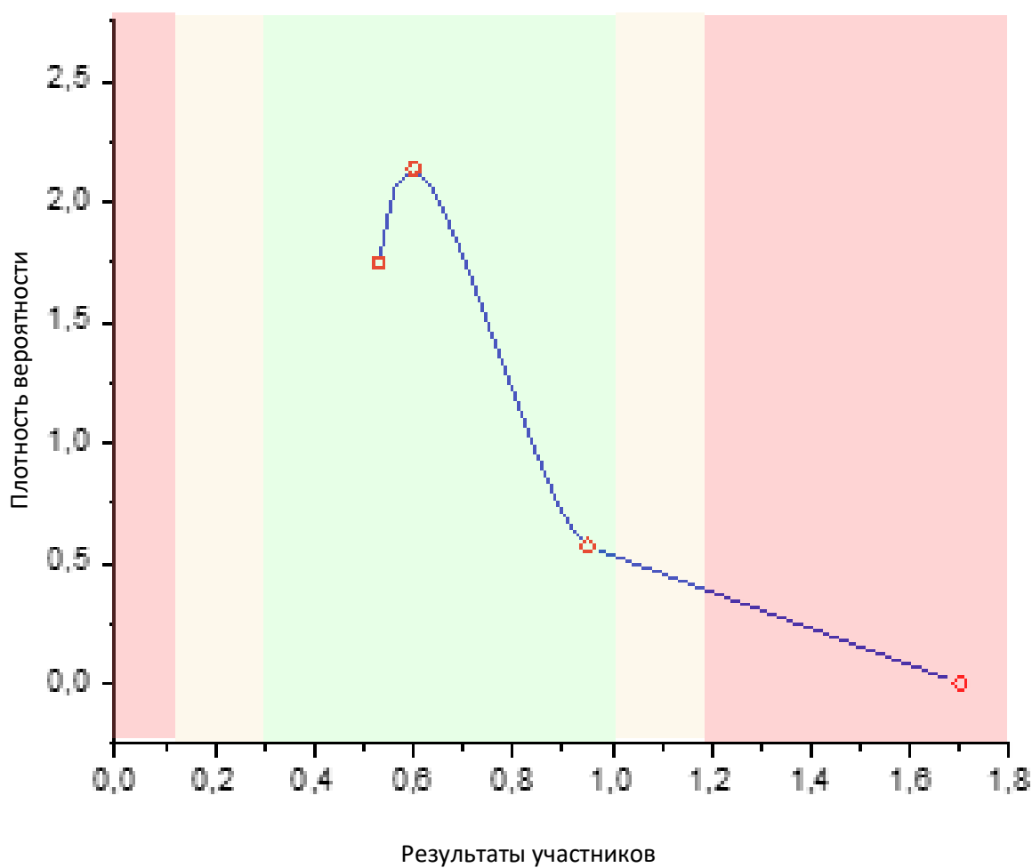
Рис. 20 Нормальное распределение по показателю «Йодное число»
